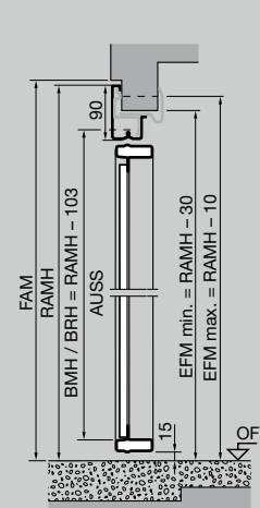
Montage par pinces sans seuil
