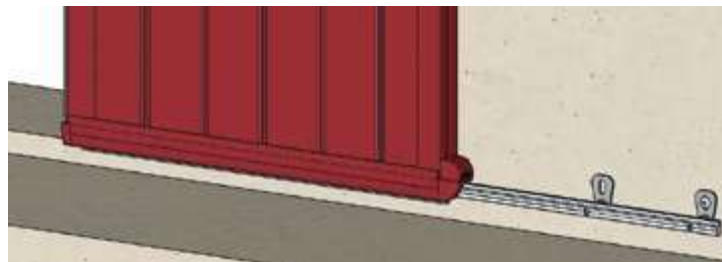
Réglette support en partie basse pour porte-fenêtre
